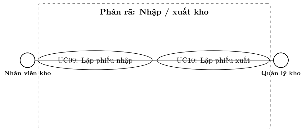
Figure 1: Use case phân rã – Lập phiếu nhập / xuất
